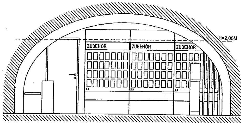
SCHNITT 2
