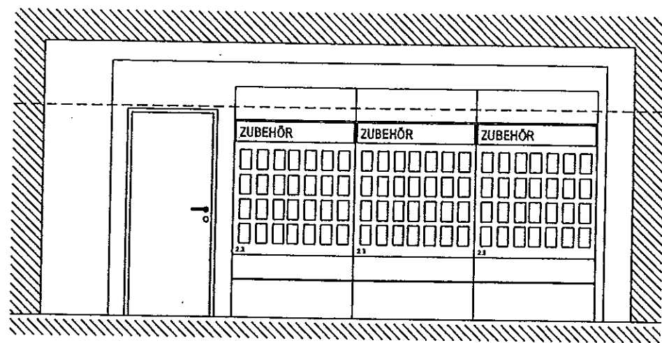
SCHNITT 3
