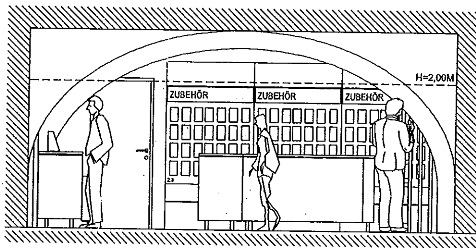
SCHNITT 1
